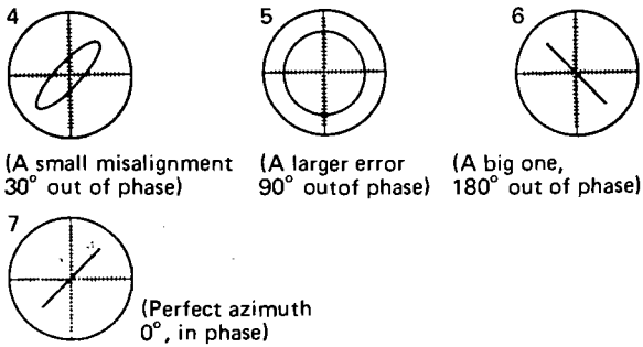
Fig. 19 Phase Shift
