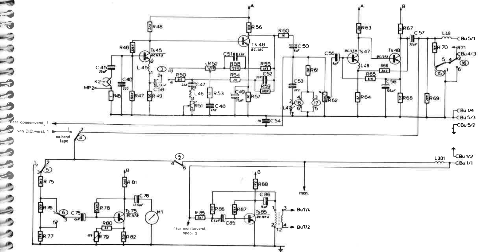
Fig. 39. Waergeefversterker in stand weergeven 19 cm/s
