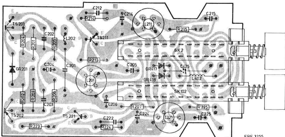
Fig. 34. Oscillator.
