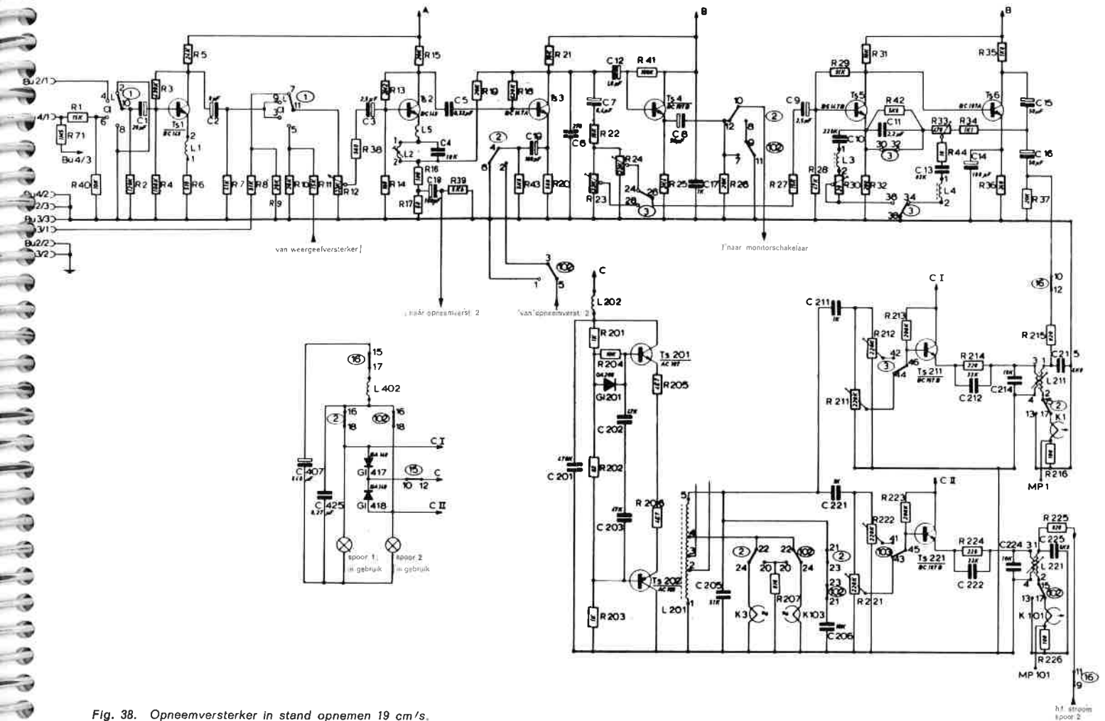
Fig. 38. Opneemversterker in stand opneemen 19 cm/s.
