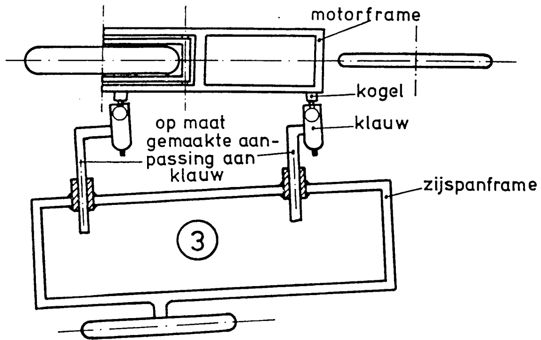
Afbeelding 34: aanpassingen klauw
