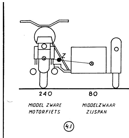
Afbeelding 4: zwaartepunt zijspan
