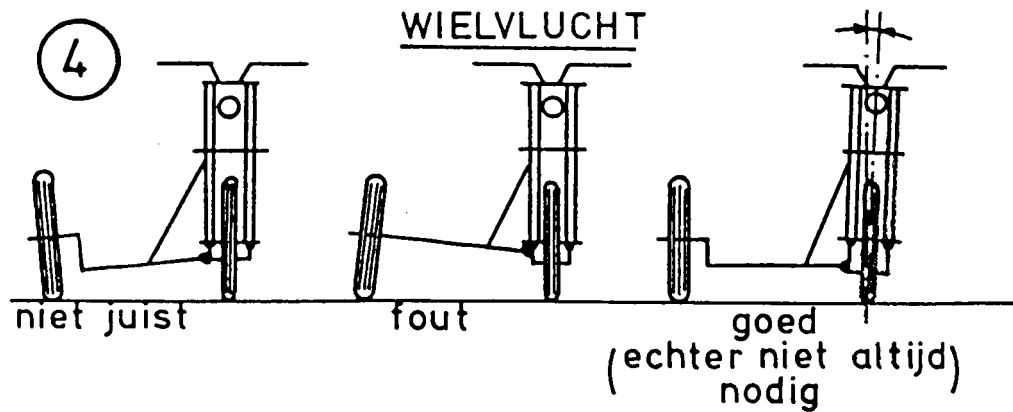
Afbeelding 37: wielvlucht
