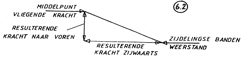
Afbeelding 16: bovenaanzicht krachten linkerbocht
