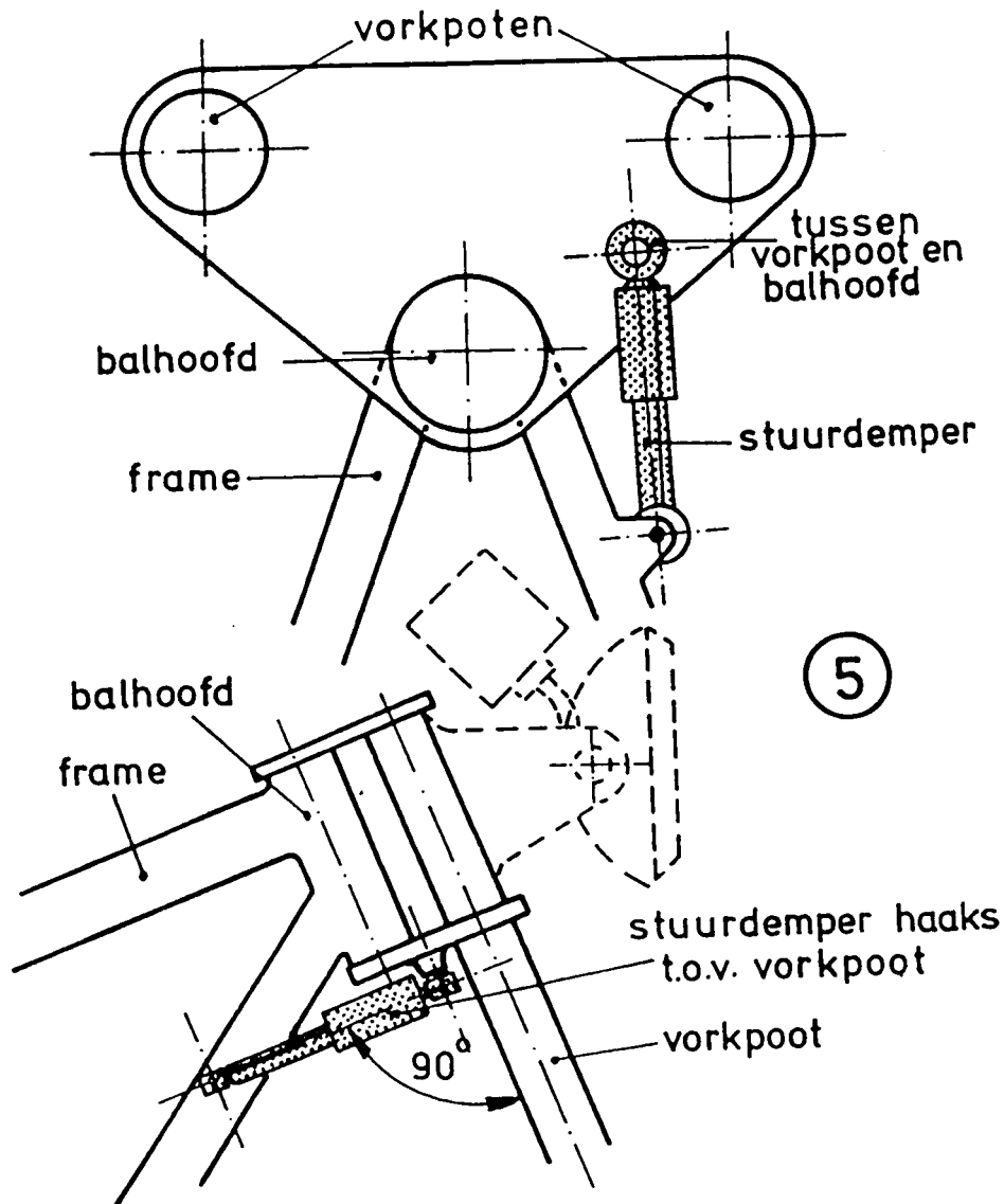
Afbeelding 36: plaatsing stuurdemper
