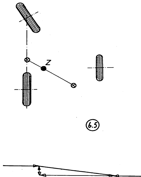
Afbeelding 19: zwaartepunt met extra belasting
